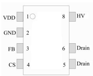
SOP-7 俯视图
